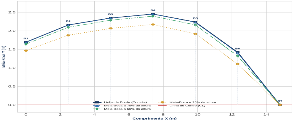
PLANO DE MEIAS-BOCAS (HALF-BREADTH PLAN)
