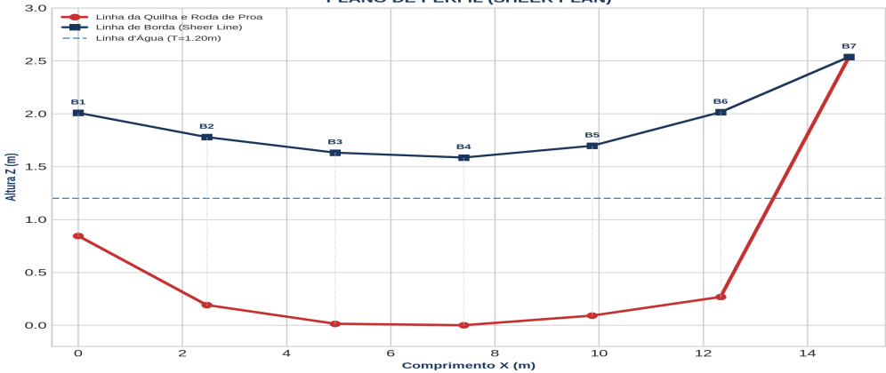
PLANO DE PERFIL (SHEER PLAN)
