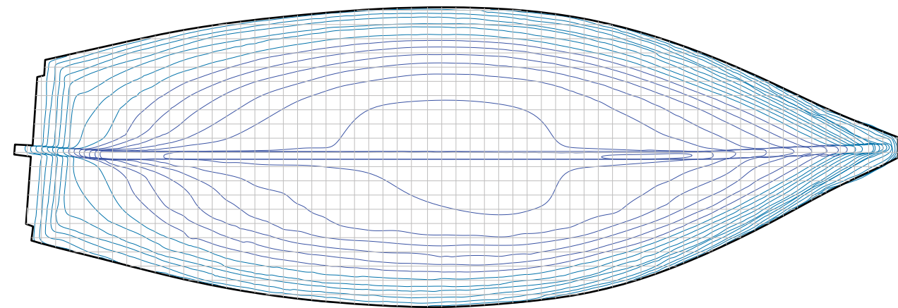
PLANO DE LINHAS D'ÁGUA
